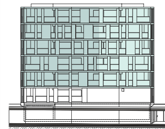
Façade SUD - EST
